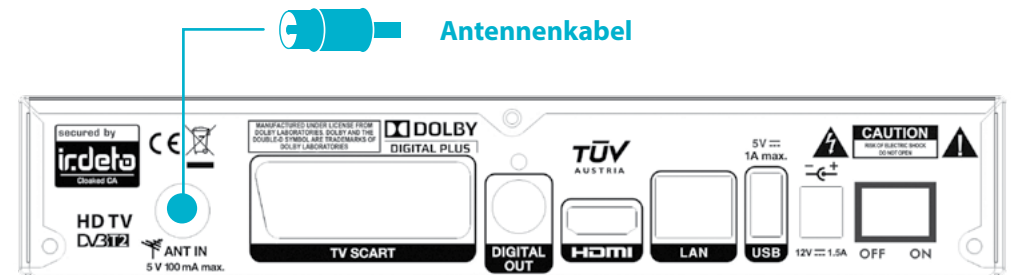
Abbildung 7: ANT IN – Eingang für das Antennenkabel
