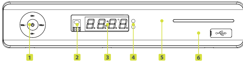
Abbildung 1: Vorderseite der Box T5213PVR
