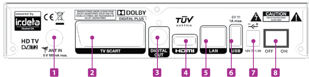
Abbildung 2: Rückseite der Box T5213PVR
