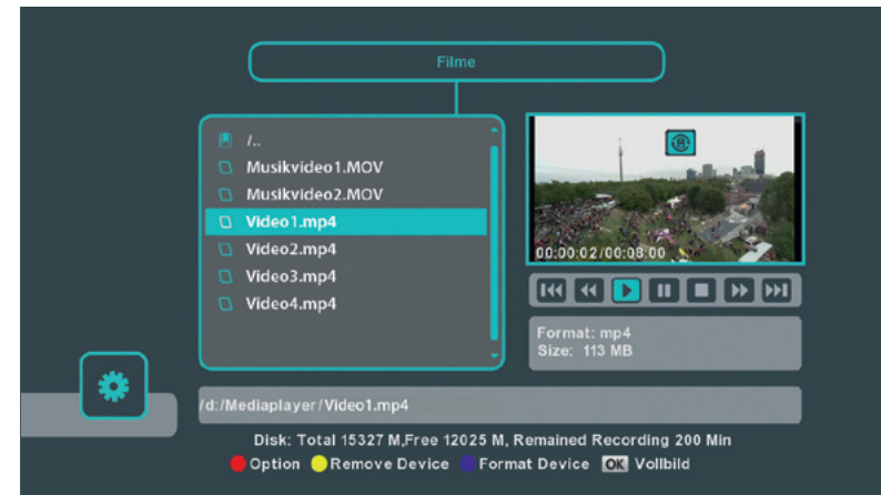
Abbildung 19: Multimedia-Player
