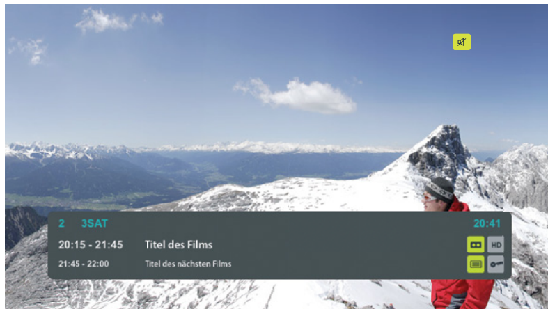
Abbildung 11: Informationsleiste
